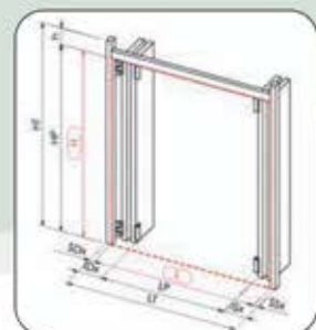
Vista isometrica Posa interna
